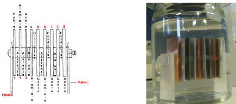
Figura 1: Disposición de los metales en el portamuestras para ensayos de corrosión. En las posiciones 1, 2 y 3 estudiaremos el comportamiento de Al, acero y cobre aislados, sin formar pares galvánicos. Entre las posiciones 4 y 5 formaremos un par galvánico Al-Cu; entre la 6 y 7 Al-acero y entre la 8 y la 9 formaremos el par Cu-Acero.
